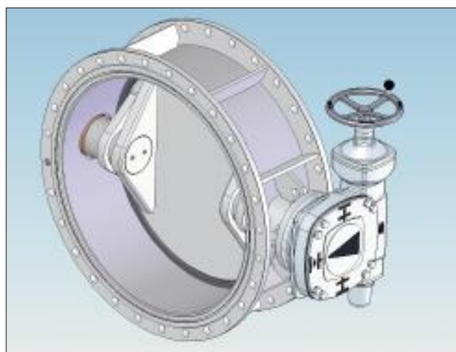
Fig. 6 Manual actuation
