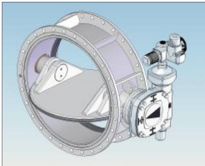
Fig. 7 Motor actuator
