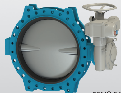
GEMÜ C488
